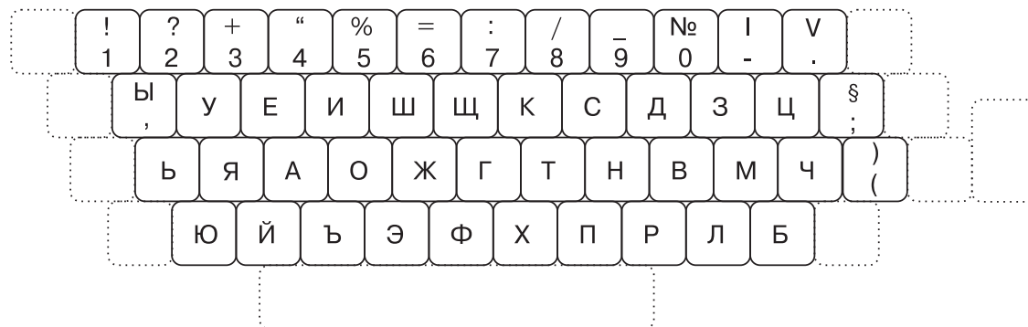
Фигура 5 Схема на клавиатурна подредба за пишещи машини с 46 буквено-цифрови клавиша
